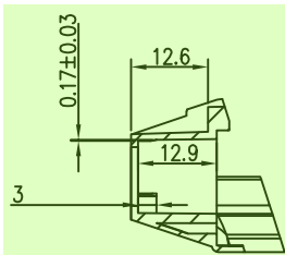
SECTION A-A5
